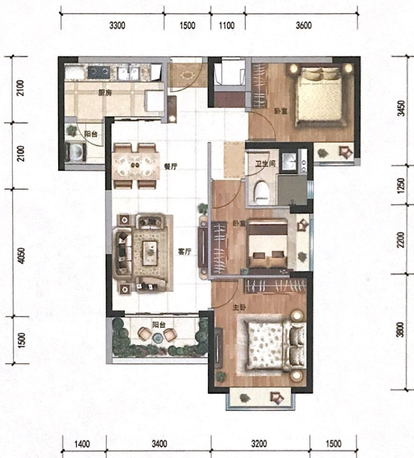
1、10、12号楼标准层
